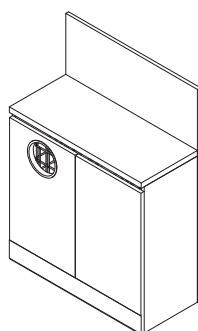
6 50842 MODULO RECICLO 80 RECYCLING MODULE 80 ↑ 1130 mm ↗ 400 mm → 800 mm
