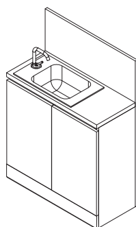
4 50832 MODULO LAVABO 80 WASHBASIN MODULE ↑ 1130 mm ↗ 400 mm → 800 mm
